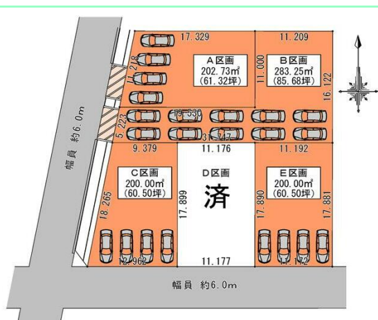
全体区画図 全5区画の開発分譲地☆
